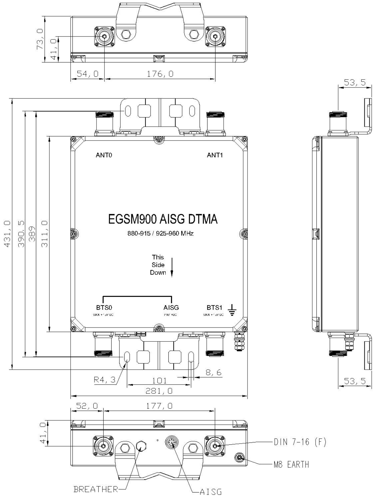
Figure 2 TY-DTMAE900-12-AISG Dimension
