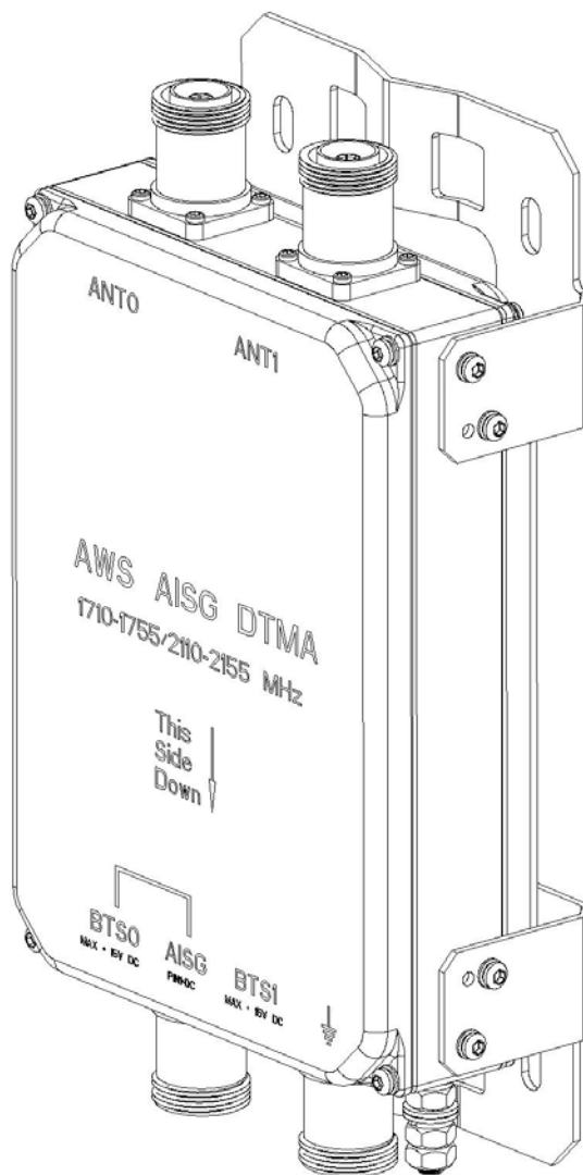
Figure 1 TY-DTMAAWS-12-AISG Twin TMA
