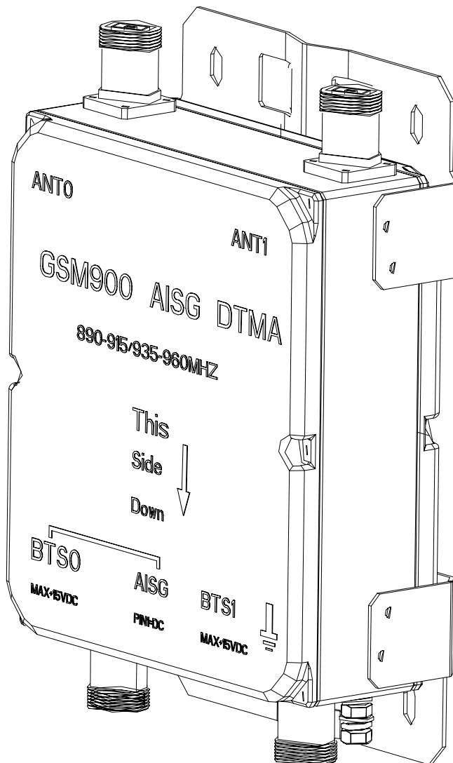
Figure 1 TY-DTMA900-12-AISG Twin TMA
