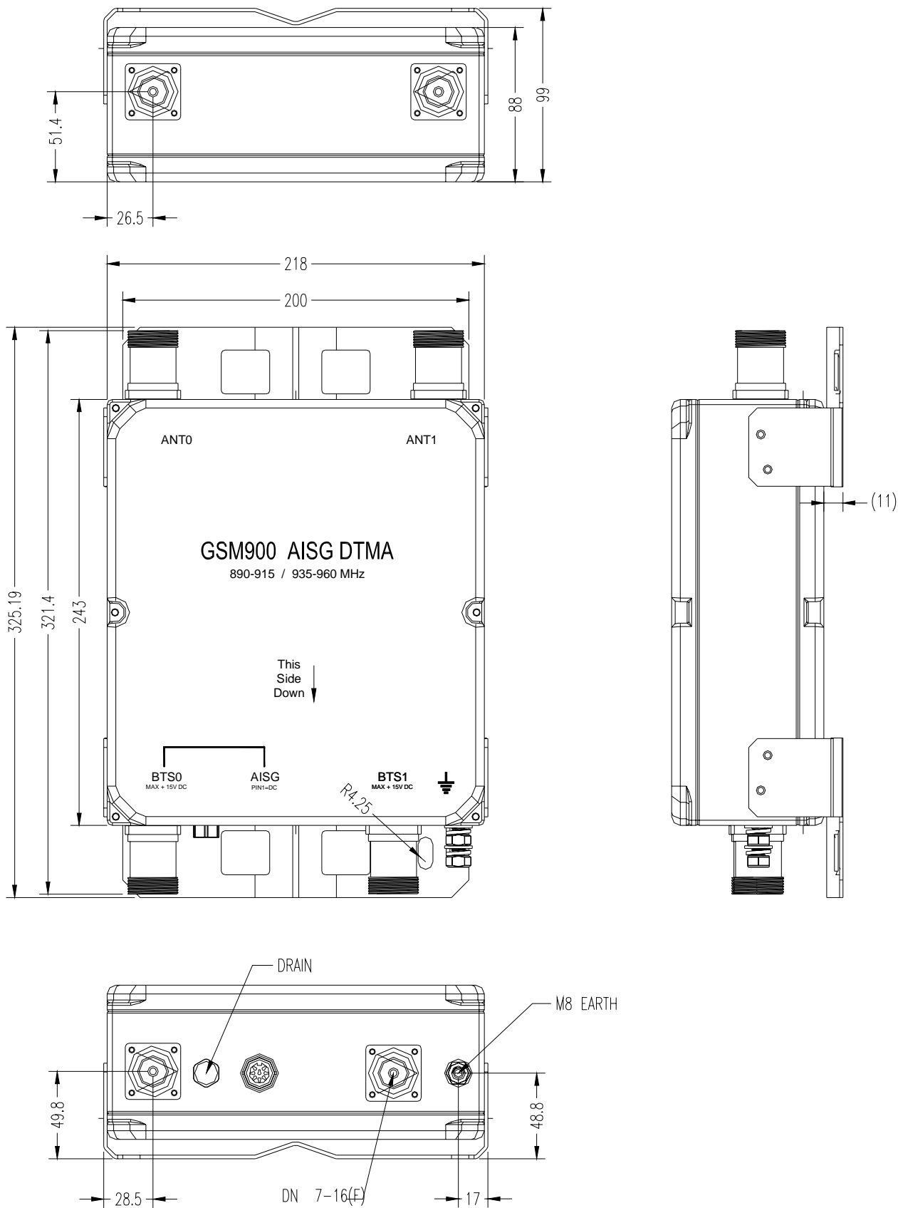
Figure 2 TY-DTMA900-12-AISG Dimension
