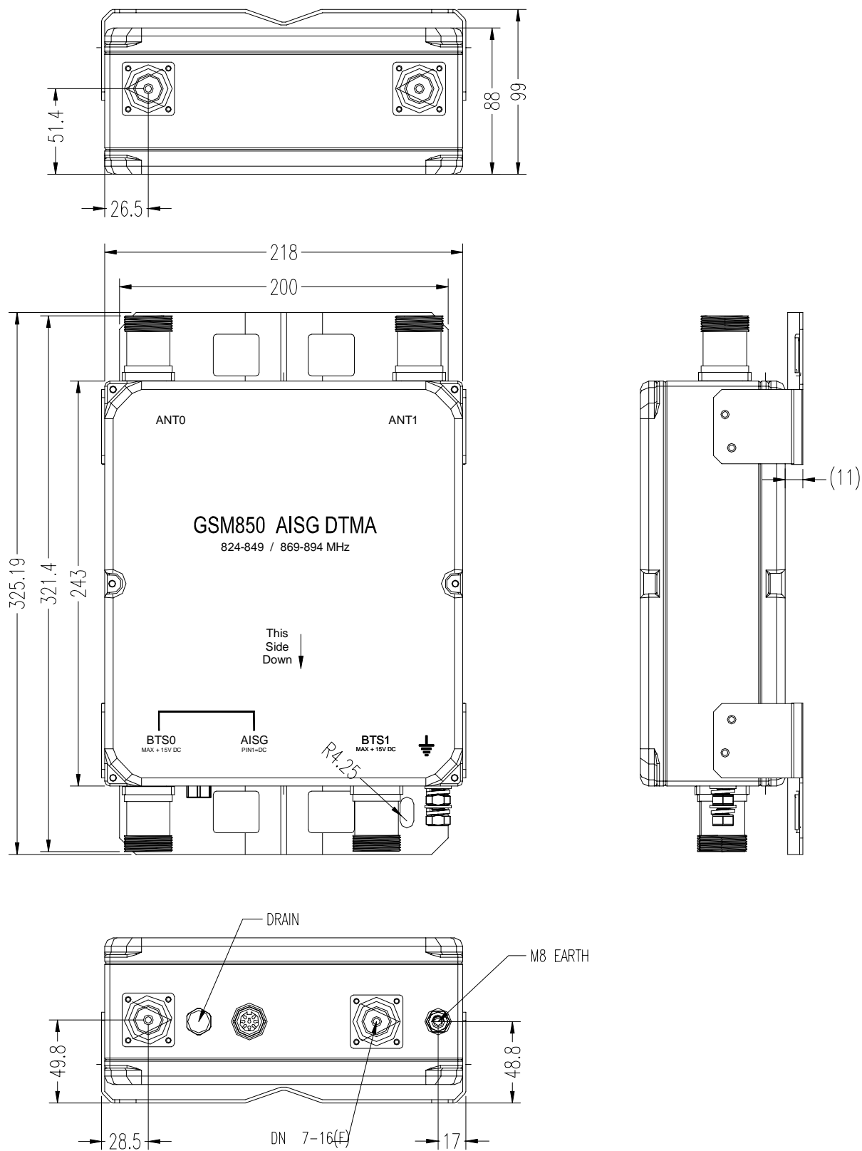
Figure 2 TY-DTMA850-12-AISG Dimension
