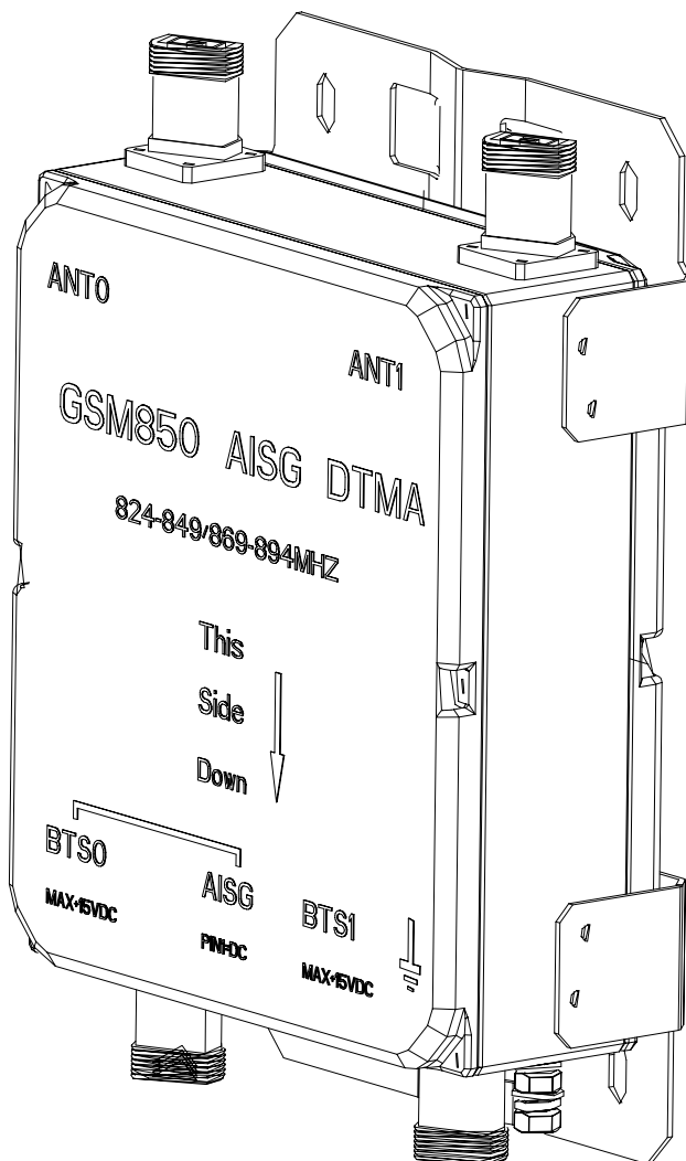
Figure 1 TY-DTMA850-12-AISG Twin TMA
