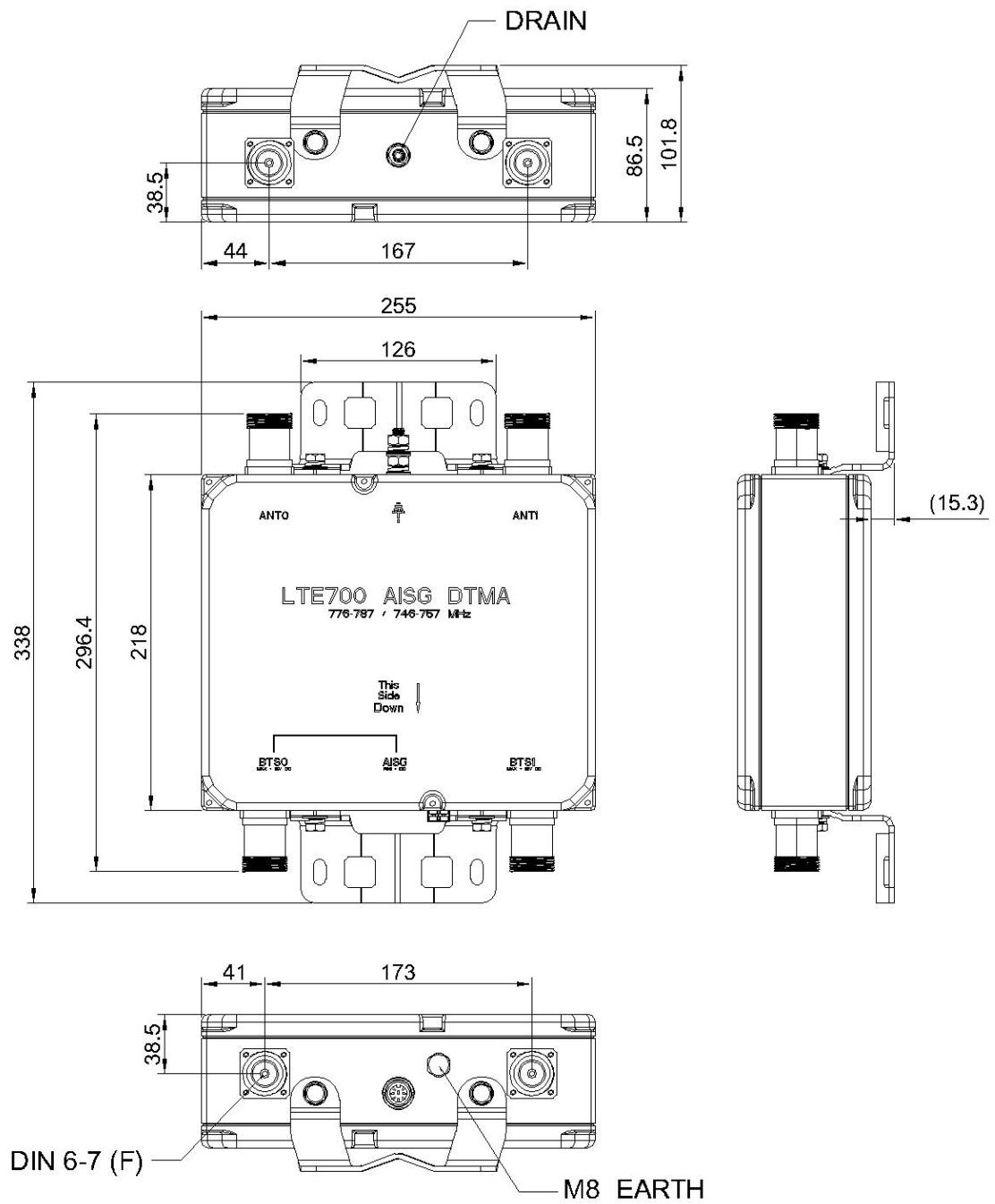
Figure 2 TY-DTMA700-12-AISG Dimension
