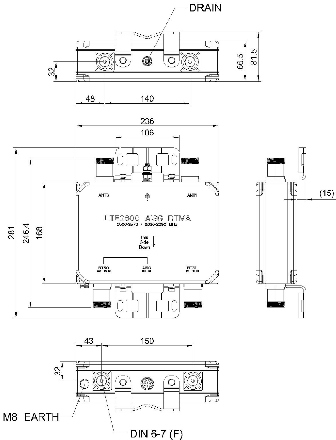
Figure 2 TYT-DTMA2600-12-AISG Dimension
